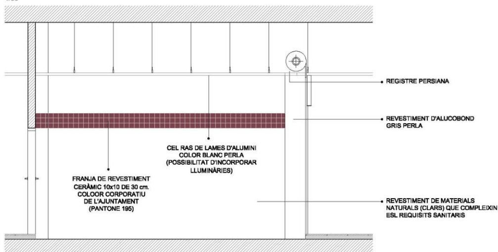
SECCIÓ PAREDES 1/50
