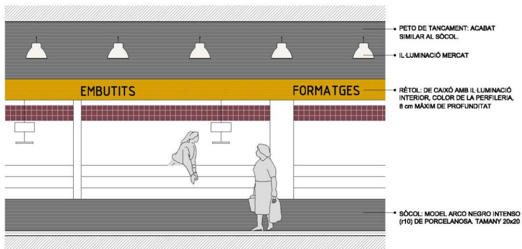
ALÇAT PAREDES 1/50
