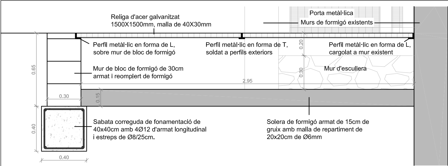
SECCIÓ A-A' DEL DETALL 1
