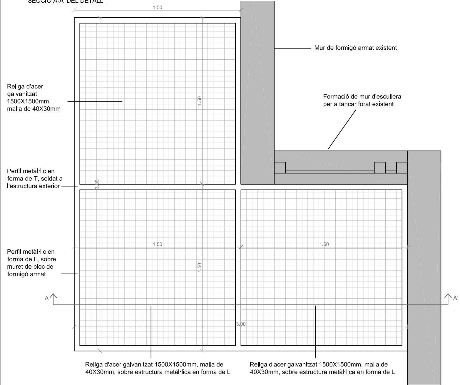
DETALL 1 : DEL NOU PERICÓ A REALITZAR A LA ZONA DEL MUR DE FORMIGÓ DE L'EXTREM SUD-OEST DEL CAMP DE FUTBOL PER TAL D'EAUAR CORRECTAMENT LES AIGUES A LA RIERA DE RIBES.
