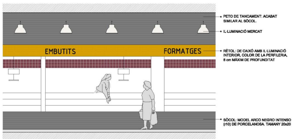
ALÇAT PARADES 1/50
