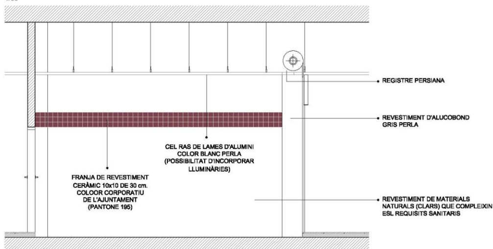
SECCIÓ PARADES 1/50
