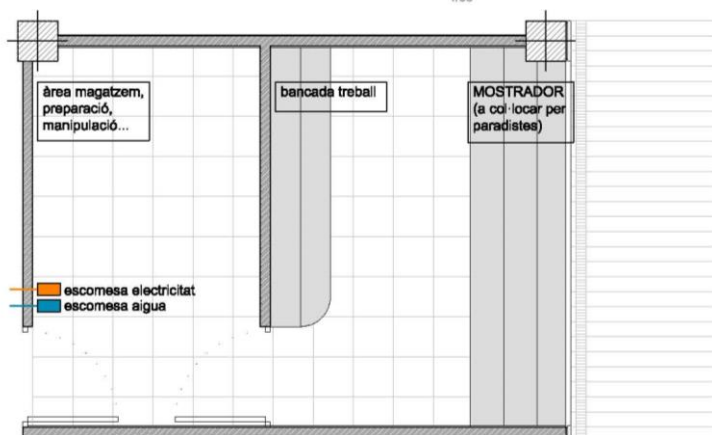
PLANTA. ESTAT INICIAL DE LES PAREDES 1/50
