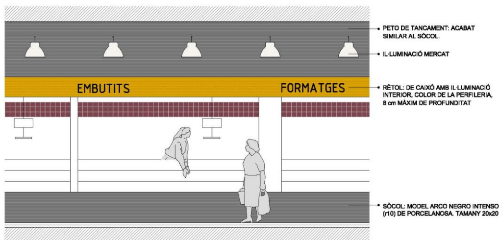
ALÇAT PARADES 1/50
