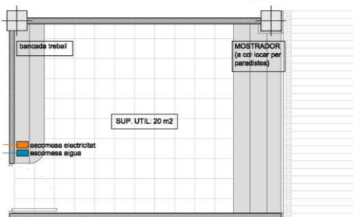
PLANTA. POSSIBLE DISTRIBUCIÓ DE LES PAREDES 1/50
