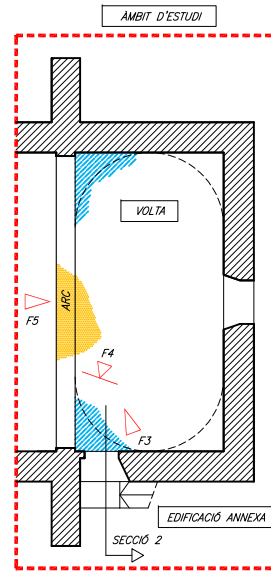
ESTRUCTURA COR ERMITA PATOLOGIES DIN A1 e:1/100
