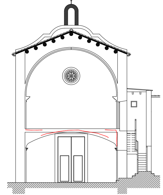
SECCIÓ 2 PATOLOGIES Arc COR DIN A1 e:1/100
