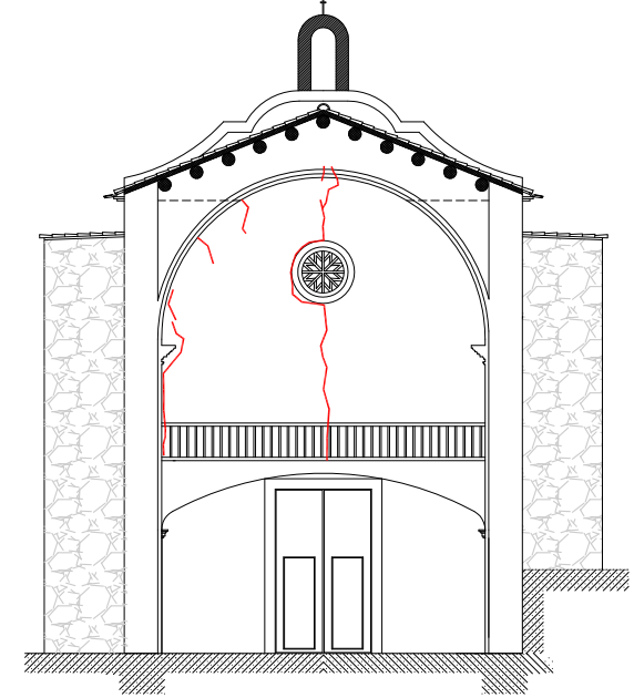
SECCIÓ 1 PATOLOGIES Façana principal DIN A1 e:1/100
