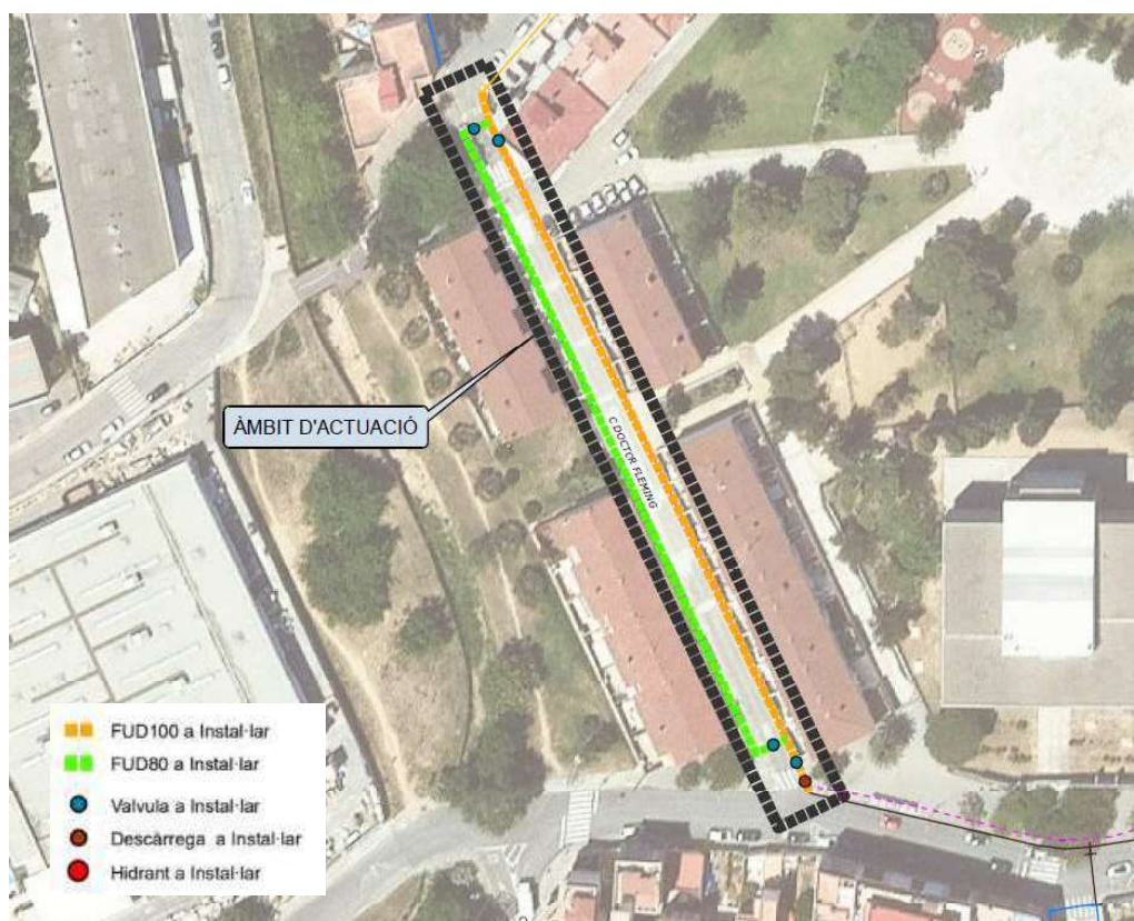
Vista en planta de la proposta d'actuació
