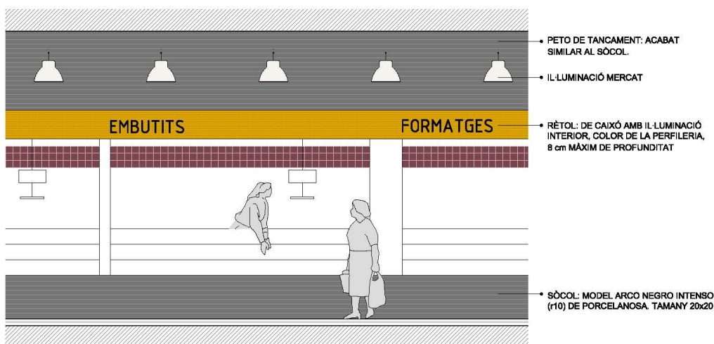
ALÇAT PARADES 1/50
