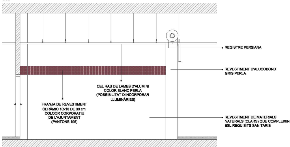
SECCIÓ PARADES 1/50
