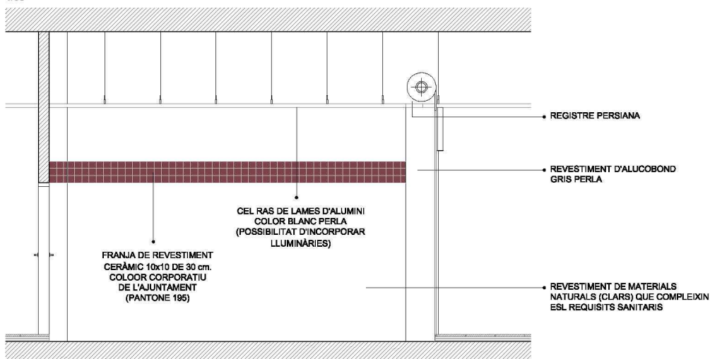
SECCIÓ PARADES 1/50
